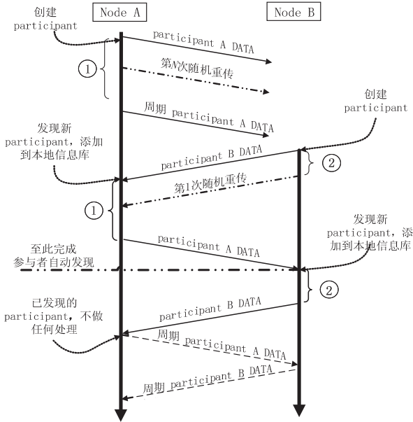
图 3 域参与者层自动发现协议控制过程
